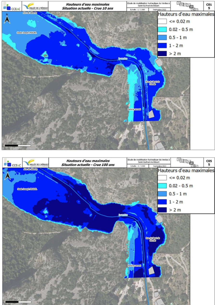
Figure 4 : Modélisation des hauteurs d'eau pour une crue décennale et centennale en situation de karst saturés
