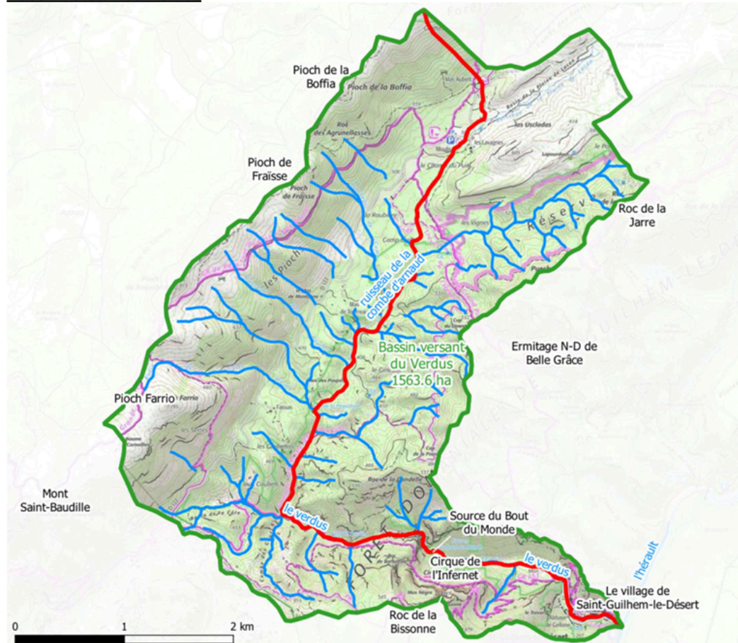
Figure 1 : Réseau hydrographique du Verdus
